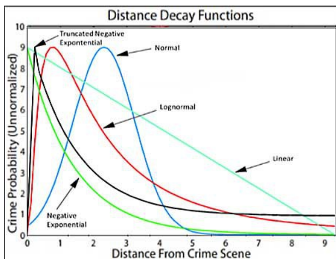
Figura 3. Muestra las funciones de Distance Decay Functions (Levine, 2007, citado en Salafranca et.al., 2020).
